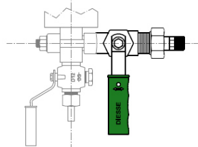
ATTACCHI AL PROCESSO RUBINETTI FILETTATI M
