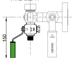
RUBINETTO DI SCARICO FILETTATO M
