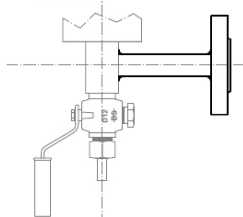
ATTACCHI AL PROCESSO FLANGIATI
