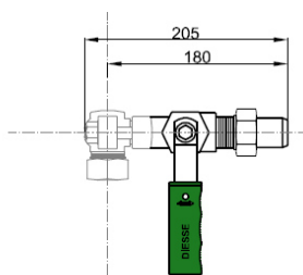
ATTACCHI AL PROCESSO RUBINETTI BW
