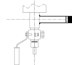
ATTACCHI AL PROCESSO FILETTATI M
