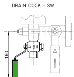
RUBINETTO DI SCARICO SW
