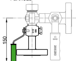
RUBINETTO DI SCARICO FLANGIATO
