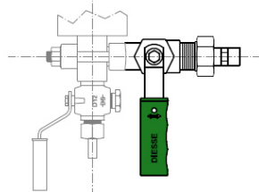
ATTACCHI AL PROCESSO RUBINETTI FILETTATI F
