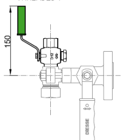
SFIATO CON TAPPO
