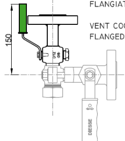
RUBINETTO DI SFIATO FLANGIATO
