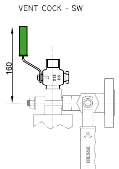
RUBINETTO DI SFIATO SW
