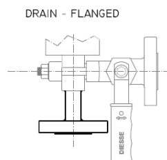
SCARICO FLANGIATO
