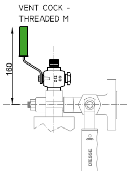
RUBINETTO DI SFIATO FILETTATO M
