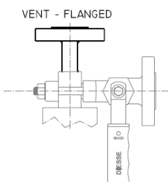
SFIATO FLANGIATO
